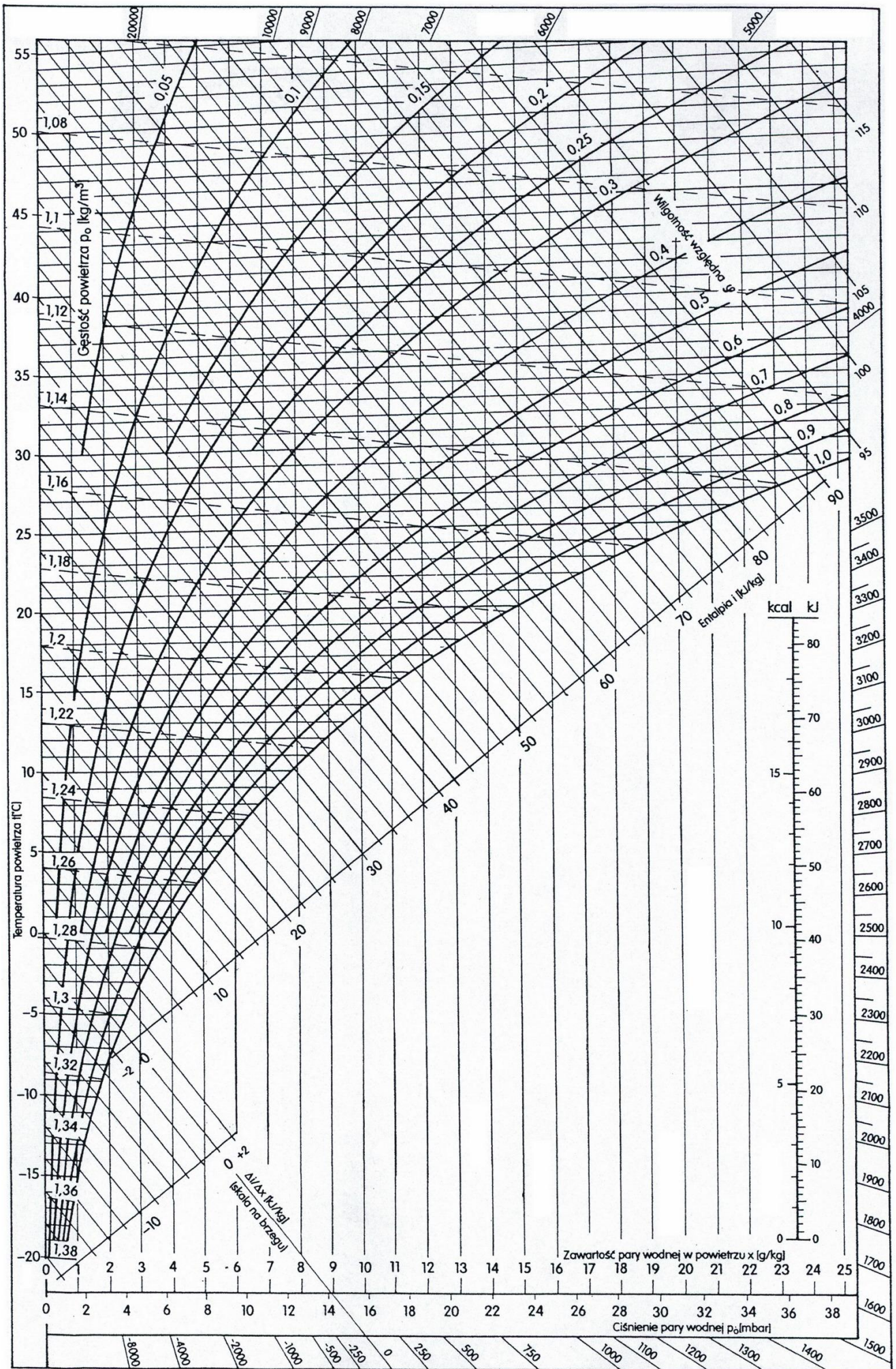
Rysunek 1: Wykres Molliera
