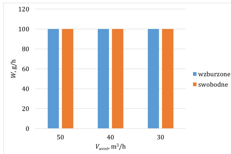
Rysunek 6: Porównanie strumieni emisji wilgoci ze swobodnego i wzburzonego zwierciadła wody dla różnych wartości strumieni powietrza wentylującego
